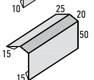
Фартук S7 пристенный в штрабу развертка 12,5 см, длина 2 м
