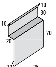
Фартук S6 пристенный накладной развертка 15 см, длина 2 м
