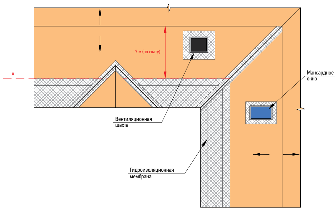
Рис. 2.22. Комбинированная гидроизоляция крыши
