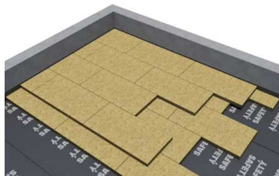
Укладка верхнего слоя теплоизоляции
