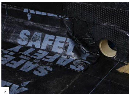
З Наплавьте первый слой кровли в соответствии с п. 4.2.1.
