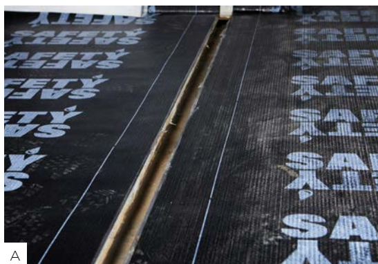
А Подведите пароизоляцию к краю шва
