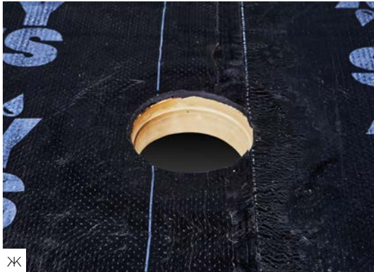
Прорежьте в первом слое кровли водосточное отверстие.
