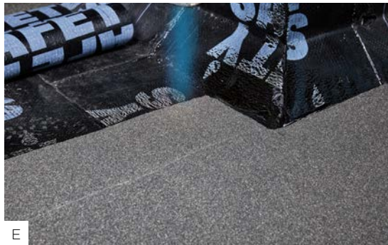
Соблюдайте нахлест смежных полотен на вертикали 80–100 мм.
