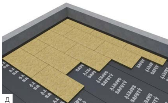
Укладка нижнего слоя теплоизоляции
