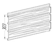
Софит сплошной
