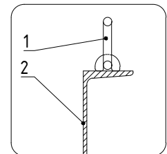
Вариант монтажа петли
