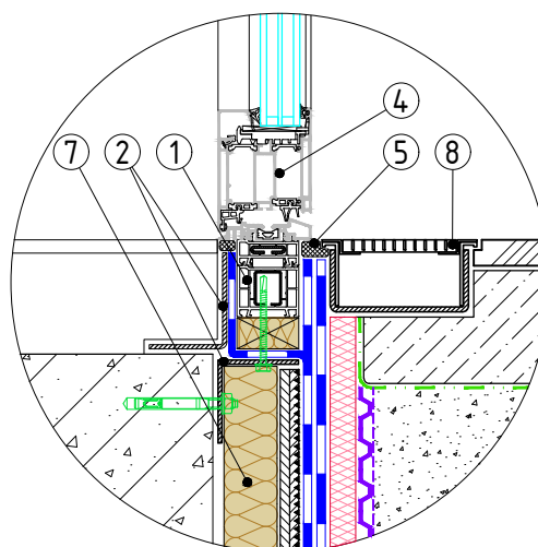
Вариант установки
